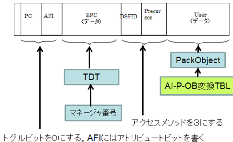
図 79 GS1 (EPC) 用(15962-a)の機能
