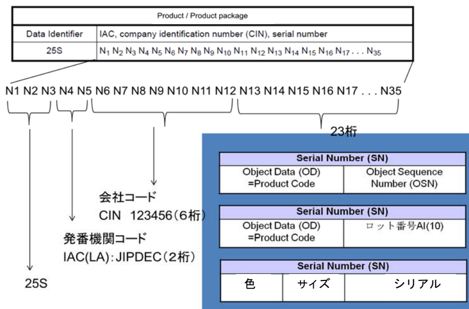
図 34 25S のマッピング方法
