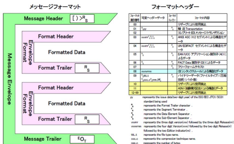
図 74 ISO/IEC 15434 のフォーマット
