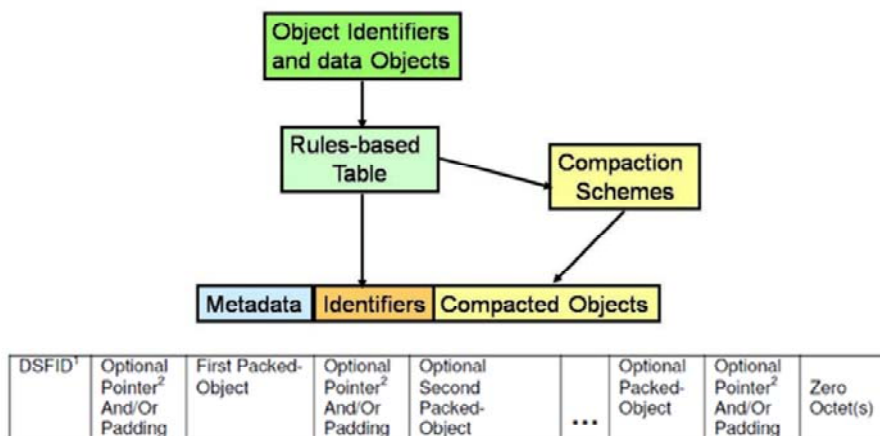
図 76 GS1 パックドオブジェクトのエンコード方法
