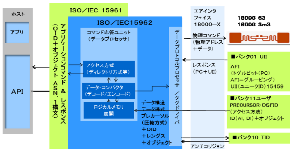
図 68 ISO データプロセッサの構造
