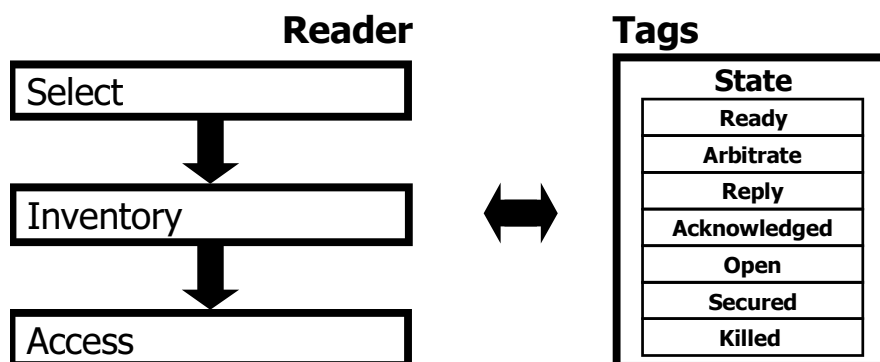
図 70 特定のタグの読み書きコマンド
