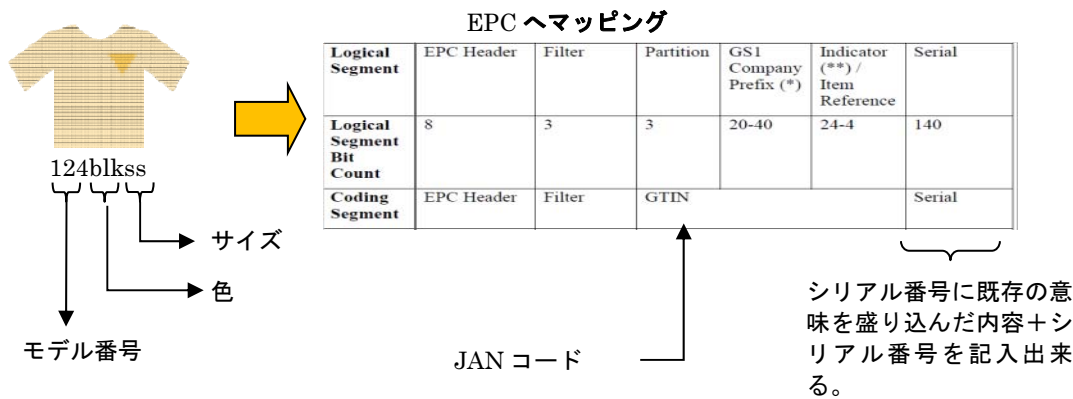
図 37 198 ビット版 EPC を使った既存コードとの共存
