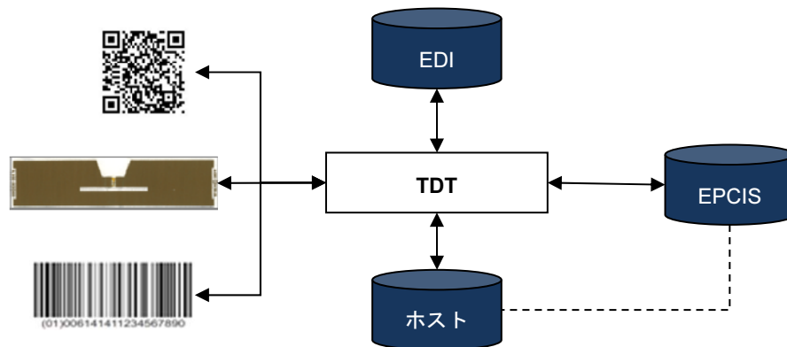
図 83 GS1 (EPC) の相互変換
