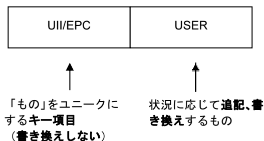
図 9 複合タグのメモリ構成
