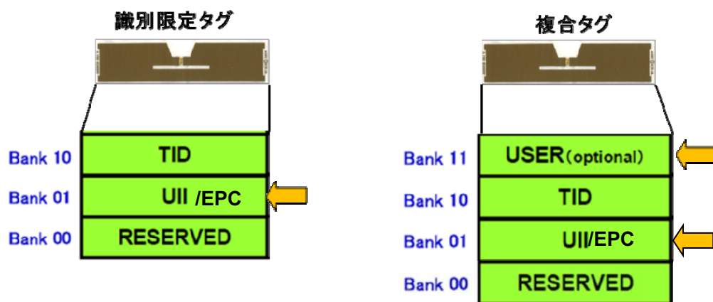
図 7 RFID のフォーマット構造
